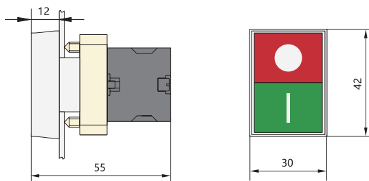
NP2-BL8325
