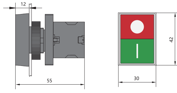
NP2-EL8325
