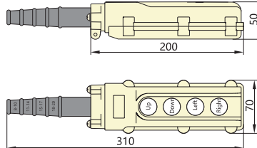
NP3-2
