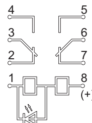
NJX12/2Z(D)
