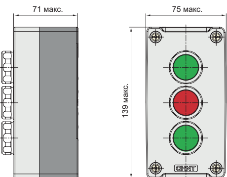
Кнопочные посты NP2-3001 ~ 3004 с 3 кнопками
