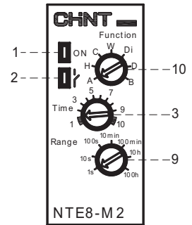
NTE8-M2
