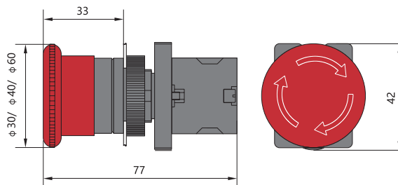
NP2-ES
