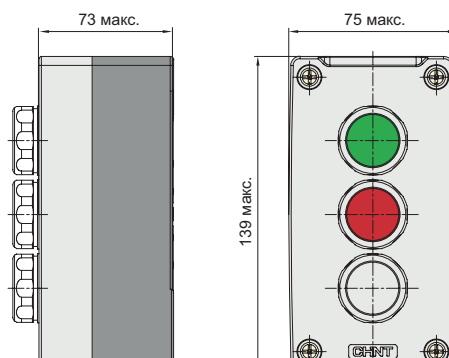
Кнопочные посты NP2-3005 ~ 3006 с 2 кнопками и индикатором
