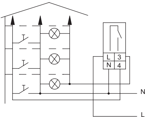
NTE8-C (3-х проводное подключение)
