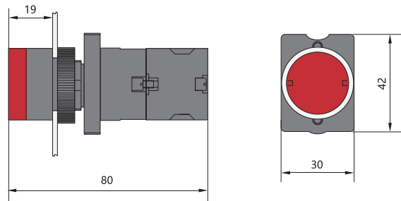
NP2-EW3
