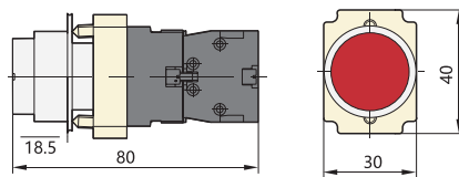
NP2-BW1
