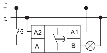
NTE8-A
