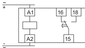
NTE8-C (4-х проводное подключение)
