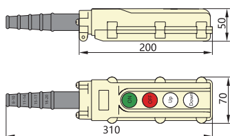
NP3-1A
