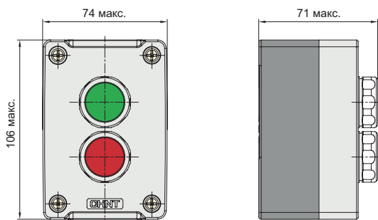
Кнопочные посты NPH1-2001 ~ 2004 с 2 кнопками
