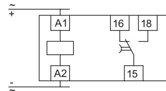
NTE8-C (4-х проводное подключение)
